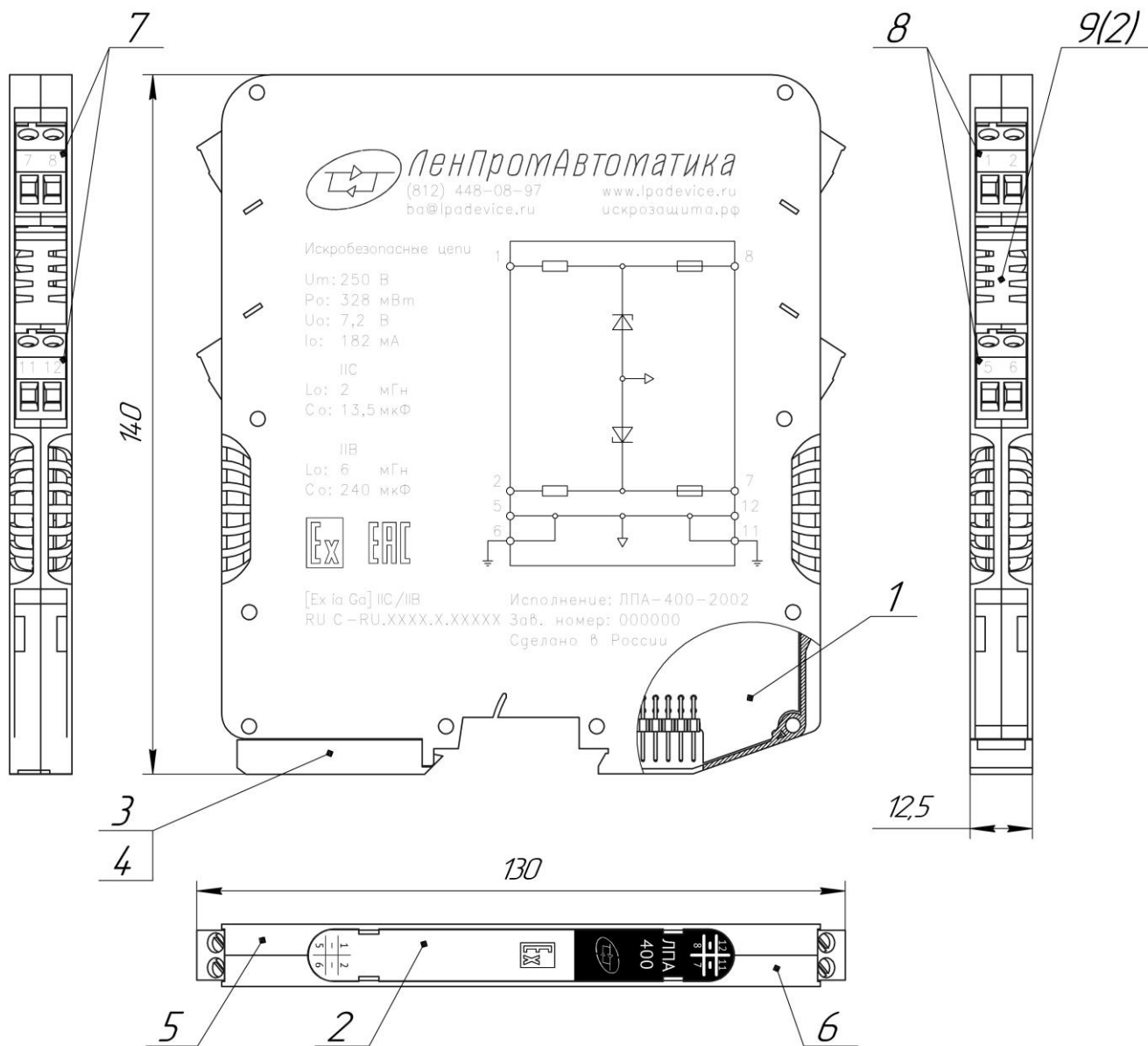
Рисунок 37 — Конструкция барьеров серии ЛПА-400
