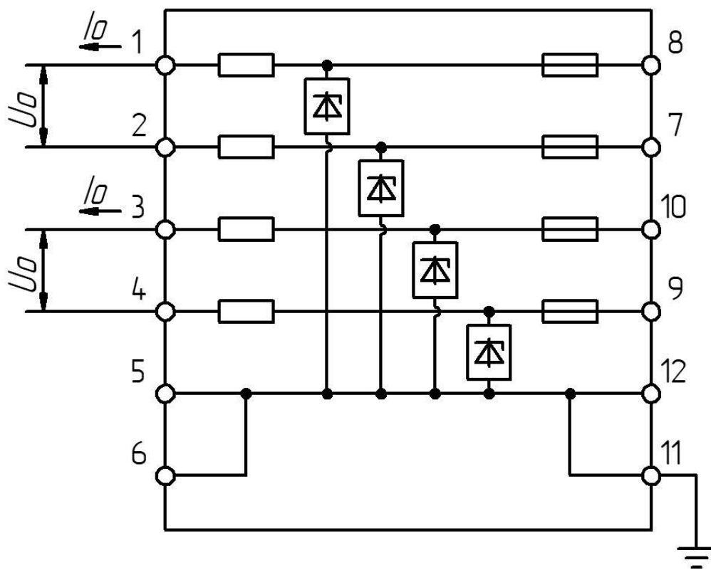
Рисунок 28 – Любые два плеча последовательно
